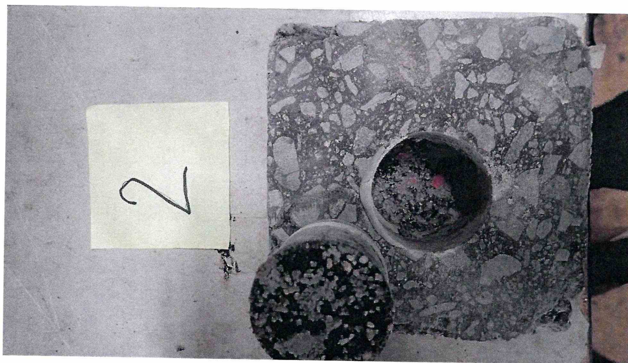
Рисунок 2 – Образец 210/4 МДС № 2, испытанный по ГОСТ Р 59180-2021. Определение прочности сцепления на отрыв при температуре -40\text{ }^{\circ}\text{C}
