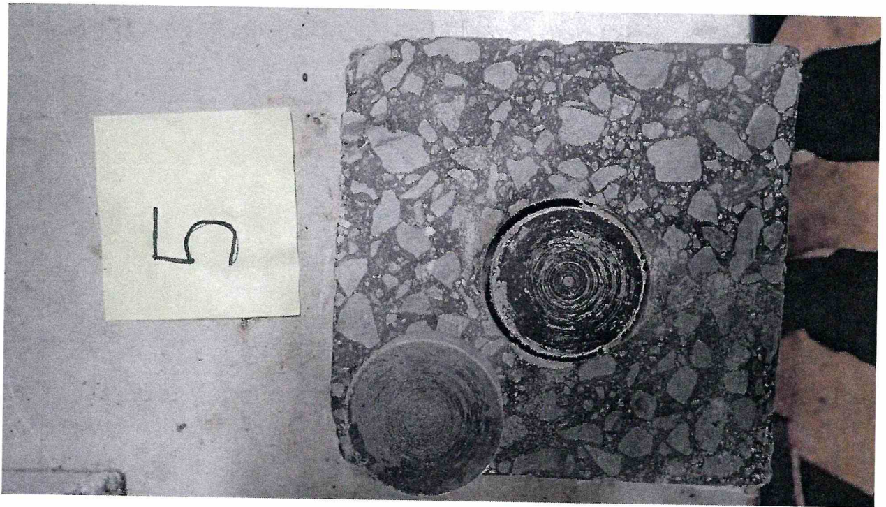
Рисунок 5 – Образец 210/4 МДС № 5, испытанный по ГОСТ Р 59180-2021. Определение прочности сцепления на отрыв при температуре -40\text{ }^{\circ}\text{C}
