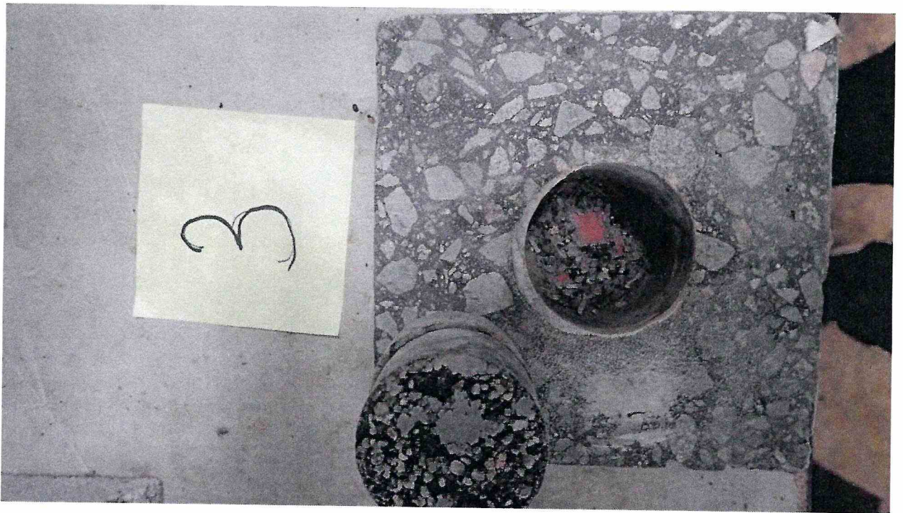
Рисунок 3 – Образец 210/4 МДС № 3, испытанный по ГОСТ Р 59180-2021. Определение прочности сцепления на отрыв при температуре -40\text{ }^{\circ}\text{C}
