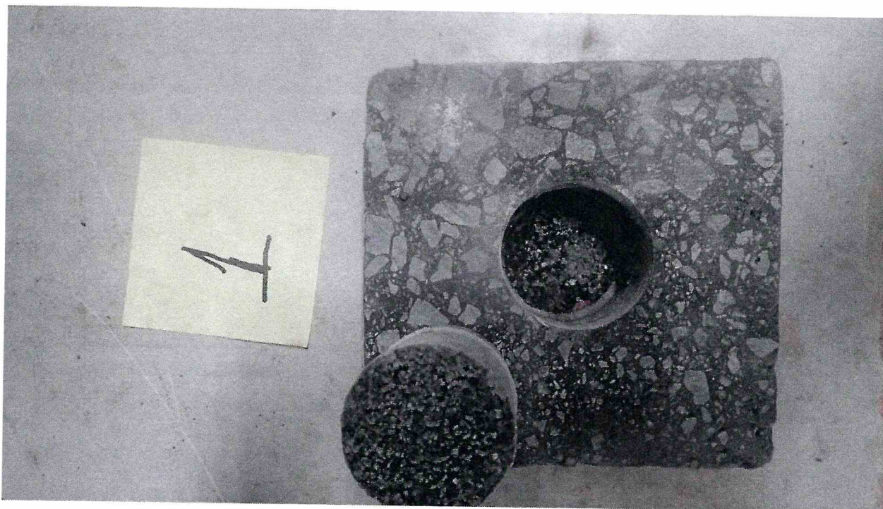
Рисунок 1 – Образец 210/4 МДС № 1, испытанный по ГОСТ Р 59180-2021. Определение прочности сцепления на отрыв при температуре -40\text{ }^{\circ}\text{C}
