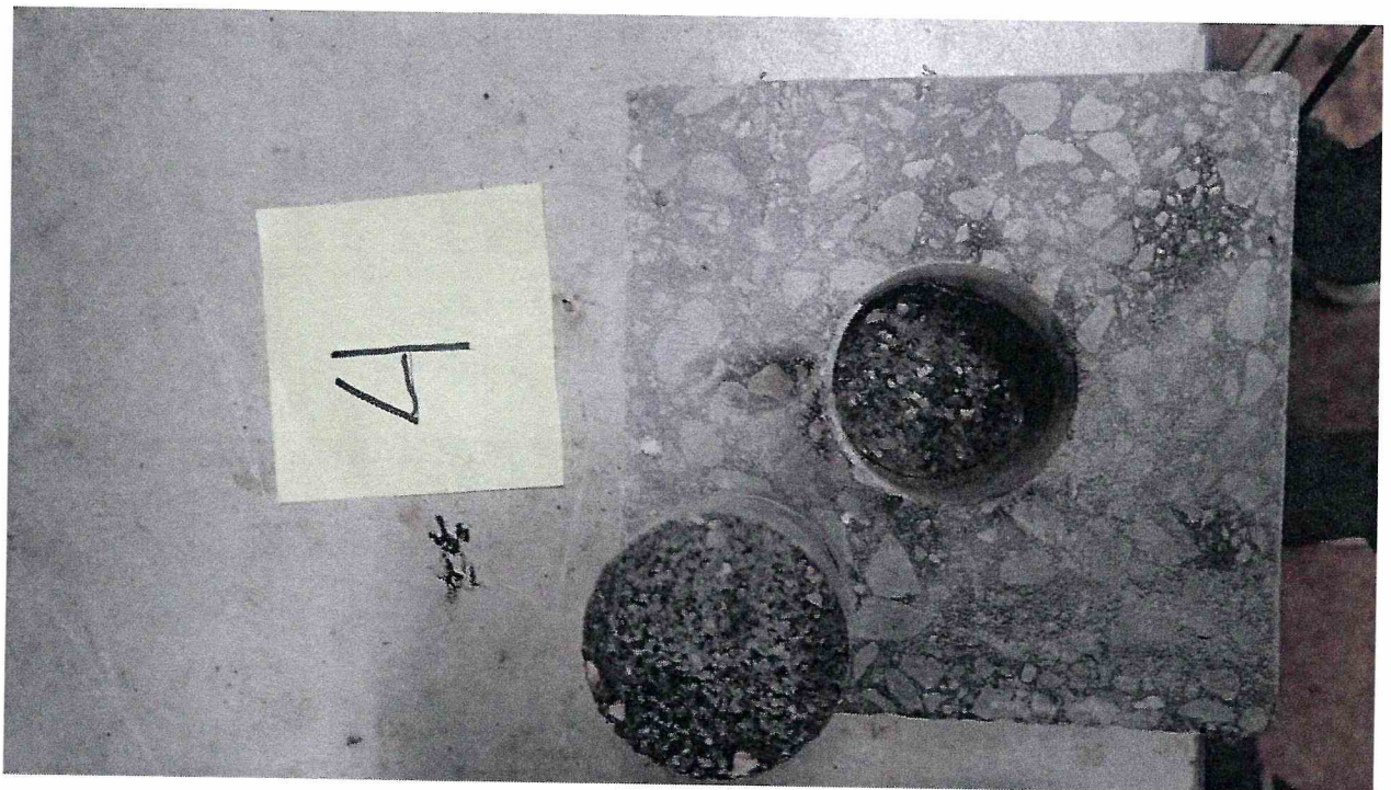
Рисунок 4 – Образец 210/4 МДС № 4, испытанный по ГОСТ Р 59180-2021. Определение прочности сцепления на отрыв при температуре -40\text{ }^{\circ}\text{C}
