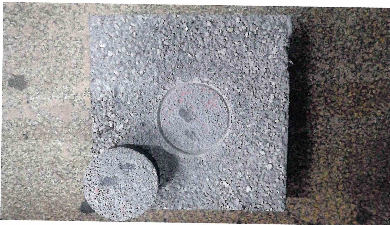
Рисунок 1 – Образец 203/3 МДС № 1, испытанный по ГОСТ Р 59180-2021. Определение прочности сцепления на отрыв при температуре 23 °С
