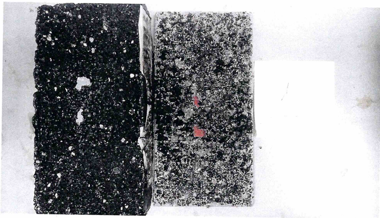
Рисунок 1 – Образец 210/1 МДС № 1, испытанный по ГОСТ Р 59180-2021. Определение прочности сцепления при сдвиге, при температуре 23 °С
