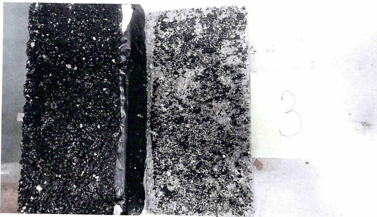
Рисунок 3 – Образец 210/1 МДС № 3, испытанный по ГОСТ Р 59180-2021. Определение прочности сцепления при сдвиге, при температуре 23 °С
