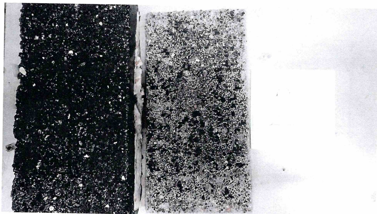
Рисунок 2 – Образец 210/1 МДС № 2, испытанный по ГОСТ Р 59180-2021. Определение прочности сцепления при сдвиге, при температуре 23 °С
