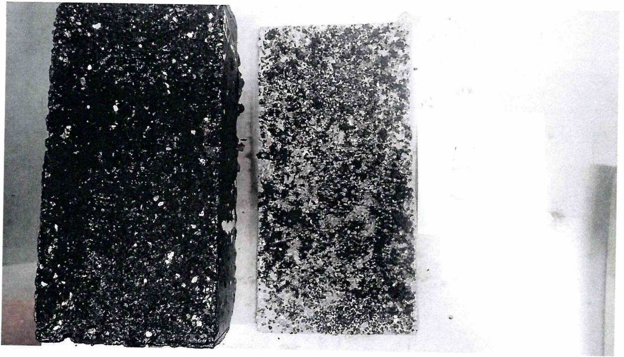
Рисунок 5 – Образец 210/1 МДС № 5, испытанный по ГОСТ Р 59180-2021. Определение прочности сцепления при сдвиге, при температуре 23 °С
