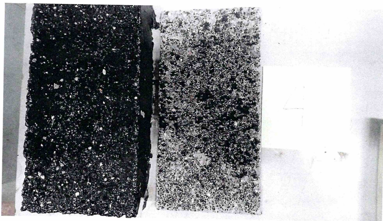
Рисунок 4 – Образец 210/1 МДС № 4, испытанный по ГОСТ Р 59180-2021. Определение прочности сцепления при сдвиге, при температуре 23 °С
