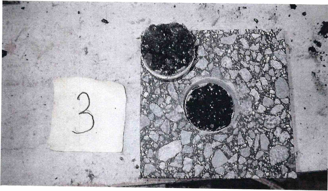
Рисунок 3 – Образец 16/4 МДС № 3, испытанный по ГОСТ Р 59180-2021. Определение прочности сцепления на отрыв при температуре 50 °С
