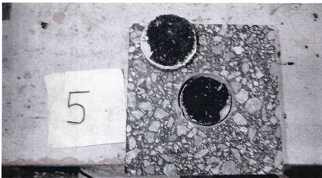
Рисунок 5 – Образец 16/4 МДС № 5, испытанный по ГОСТ Р 59180-2021. Определение прочности сцепления на отрыв при температуре 50 °С
