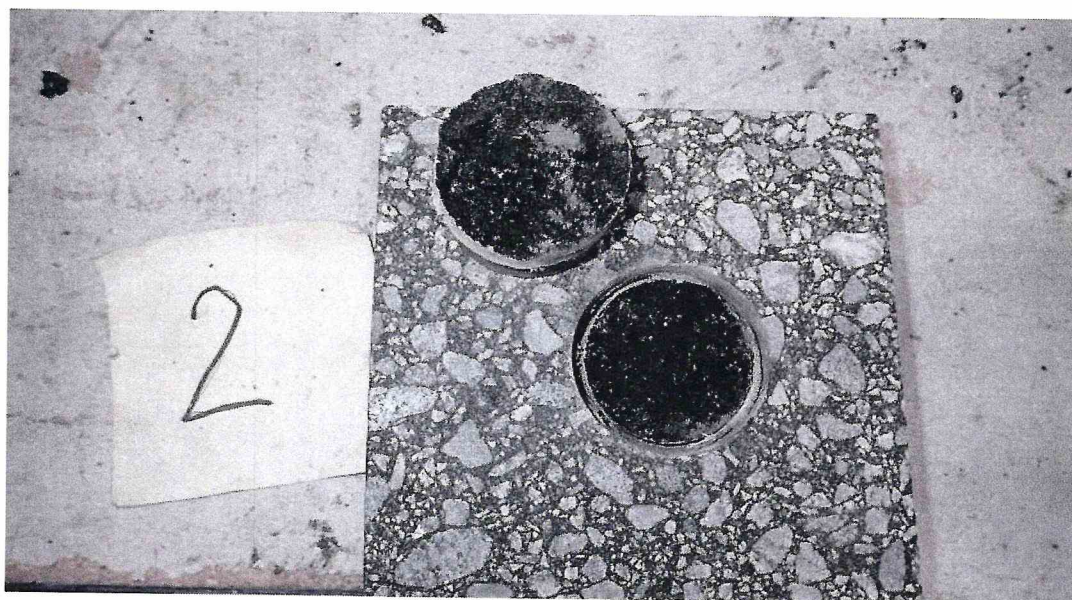
Рисунок 2 – Образец 16/4 МДС № 2, испытанный по ГОСТ Р 59180-2021. Определение прочности сцепления на отрыв при температуре 50 °С
