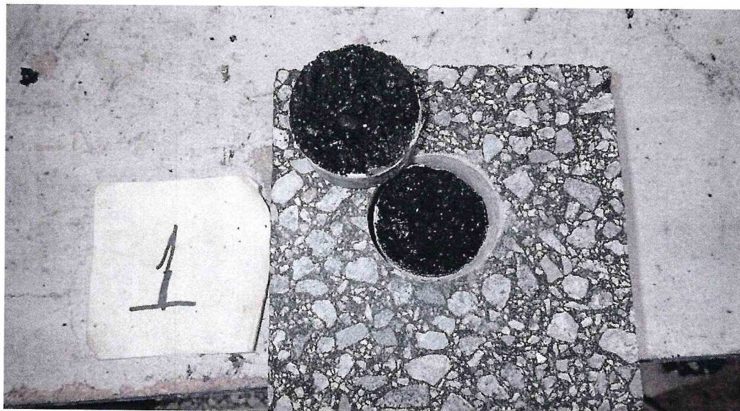
Рисунок 1 – Образец 16/4 МДС № 1, испытанный по ГОСТ Р 59180-2021. Определение прочности сцепления на отрыв при температуре 50 °С
