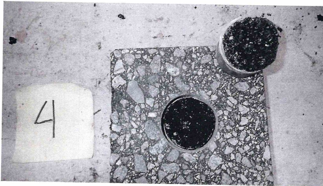
Рисунок 4 – Образец 16/4 МДС № 4, испытанный по ГОСТ Р 59180-2021. Определение прочности сцепления на отрыв при температуре 50 °С
