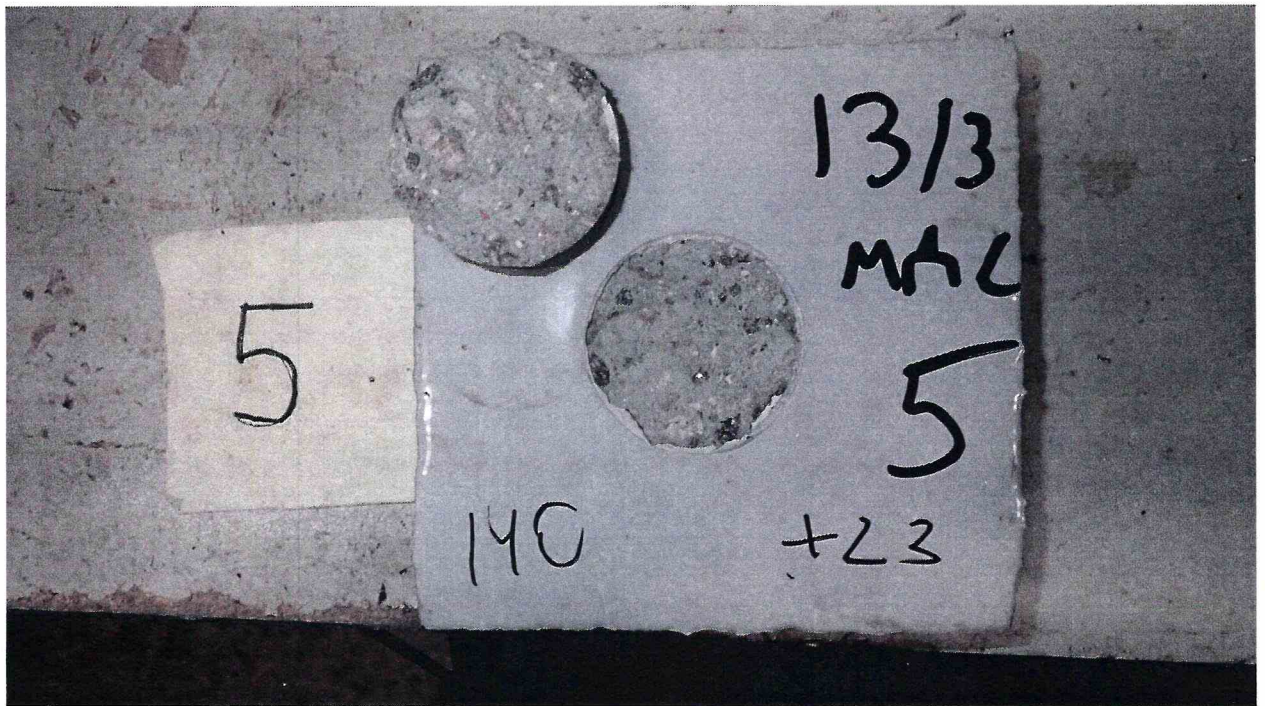
Рисунок 5 – Образец 13/3 МДС № 5, испытанный по ГОСТ Р 59180-2021. Определение прочности сцепления на отрыв при температуре 23 °С
