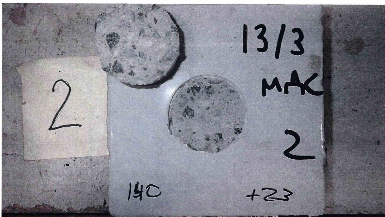
Рисунок 2 – Образец 13/3 МДС № 2, испытанный по ГОСТ Р 59180-2021. Определение прочности сцепления на отрыв при температуре 23 °С
