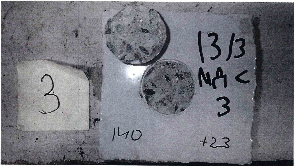
Рисунок 3 – Образец 13/3 МДС № 3, испытанный по ГОСТ Р 59180-2021. Определение прочности сцепления на отрыв при температуре 23 °С
