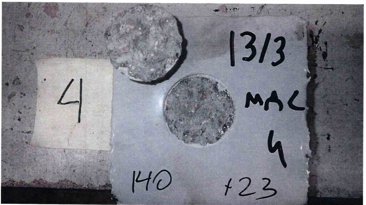
Рисунок 4 – Образец 13/3 МДС № 4, испытанный по ГОСТ Р 59180-2021. Определение прочности сцепления на отрыв при температуре 23 °С
