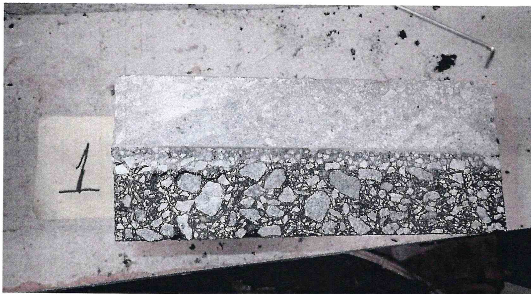
Рисунок 1 – Образец 16/1 МДС № 1, испытанный по ГОСТ Р 59180-2021. Определение прочности сцепления при сдвиге при температуре 50 °С
