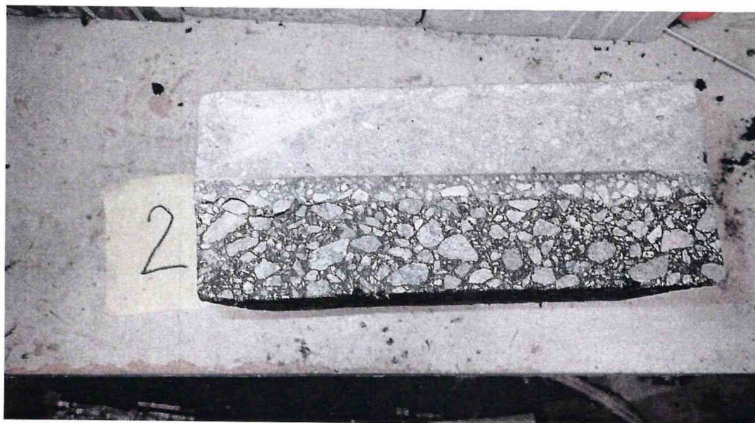
Рисунок 2 – Образец 16/1 МДС № 2, испытанный по ГОСТ Р 59180-2021. Определение прочности сцепления при сдвиге при температуре 50 °С
