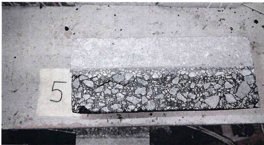
Рисунок 5 – Образец 16/1 МДС № 5, испытанный по ГОСТ Р 59180-2021. Определение прочности сцепления при сдвиге при температуре 50 °С
