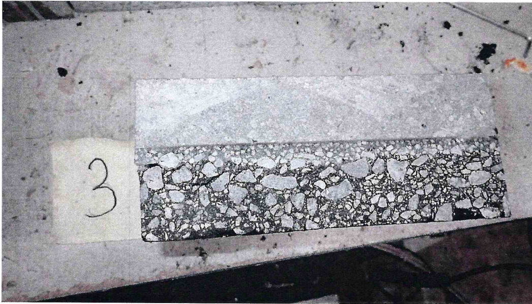
Рисунок 3 – Образец 16/1 МДС № 3, испытанный по ГОСТ Р 59180-2021. Определение прочности сцепления при сдвиге при температуре 50 °С
