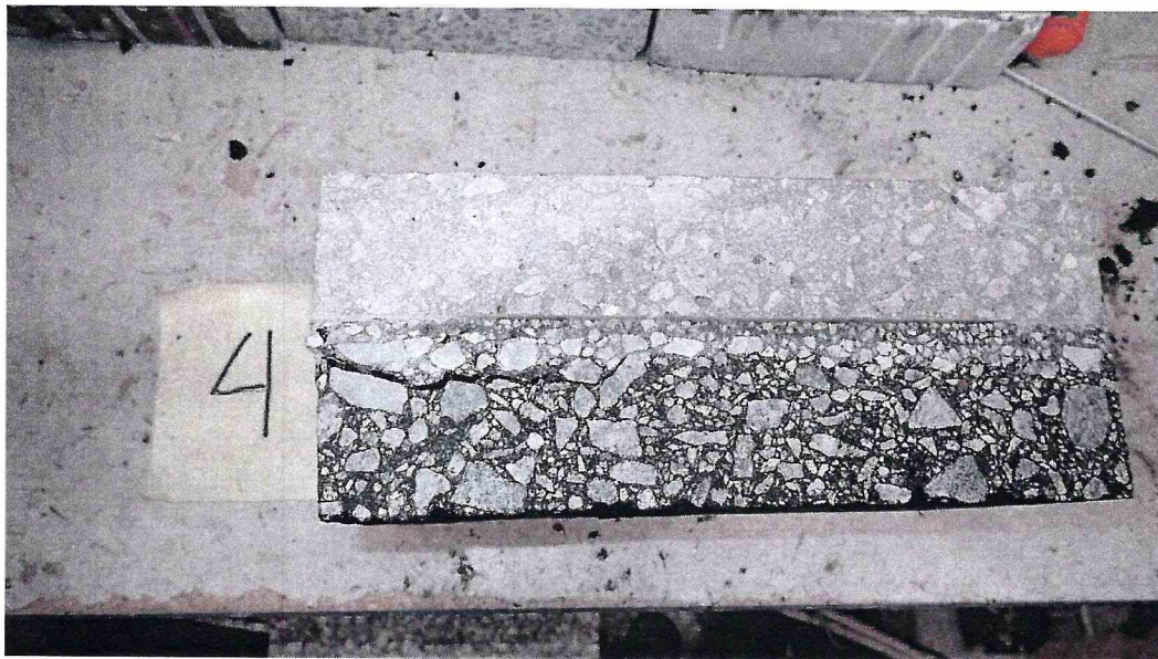
Рисунок 4 – Образец 16/1 МДС № 4, испытанный по ГОСТ Р 59180-2021. Определение прочности сцепления при сдвиге при температуре 50 °С
