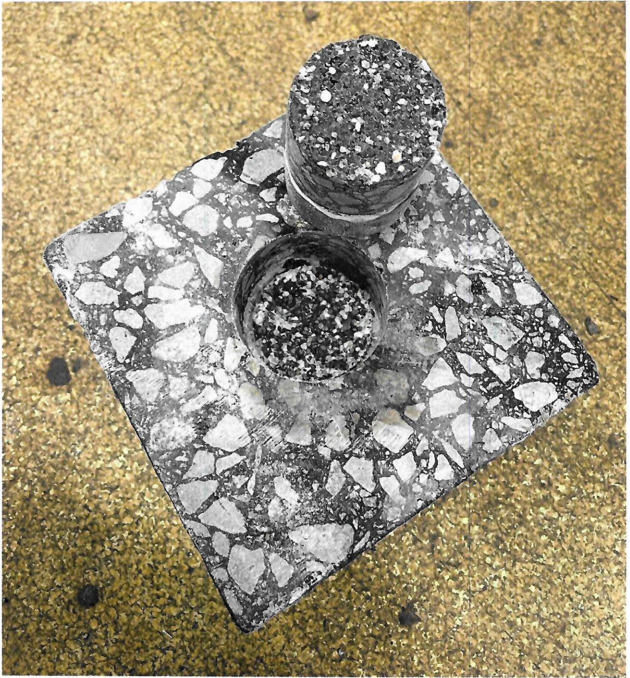
Рисунок 3 – Образец № 3 -40 МДС, испытанный по ГОСТ Р 55402-2013, ГОСТ Р 59180-2021, определение прочности сцепления на отрыв при температуре -40°C
