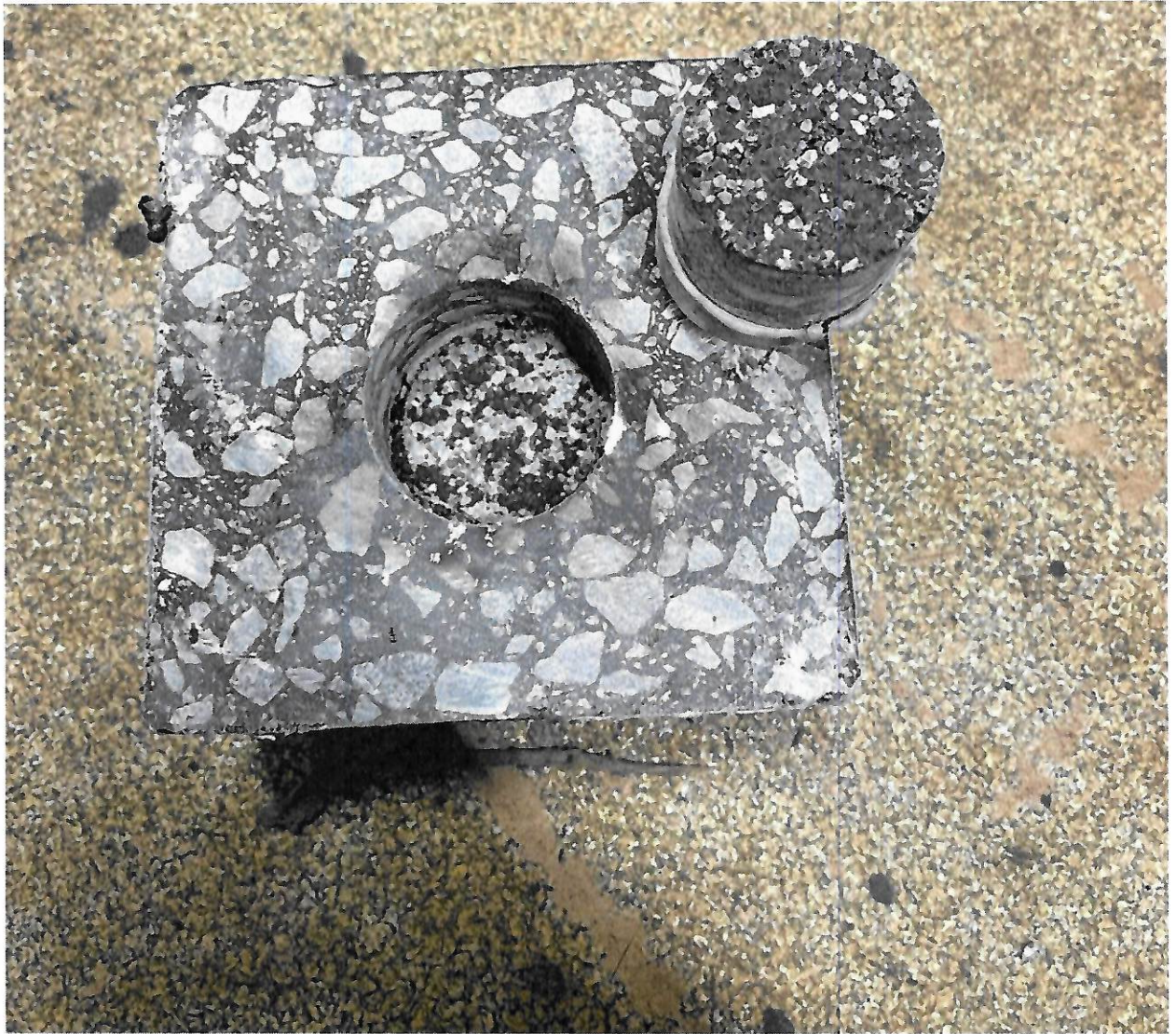
Рисунок 2 – Образец № 2 -40 МДС, испытанный по ГОСТ Р 55402-2013, ГОСТ Р 59180-2021, определение прочности сцепления на отрыв при температуре -40°С
