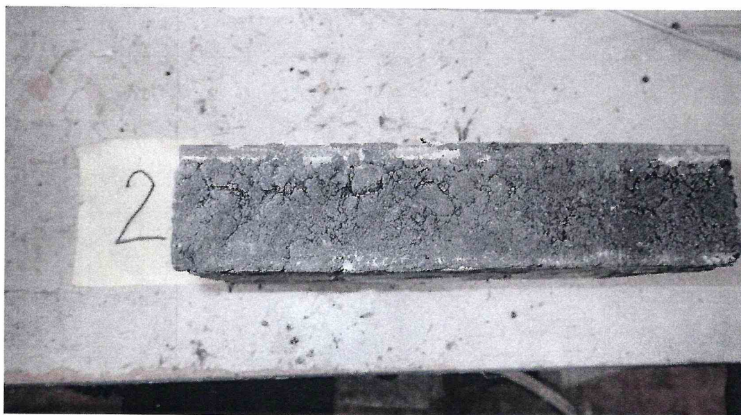
Рисунок 2 – Образец 16/7 МДС № 2, испытанный по ГОСТ Р 59180-2021. Определение прочности сцепления при сдвиге при температуре -40 °С
