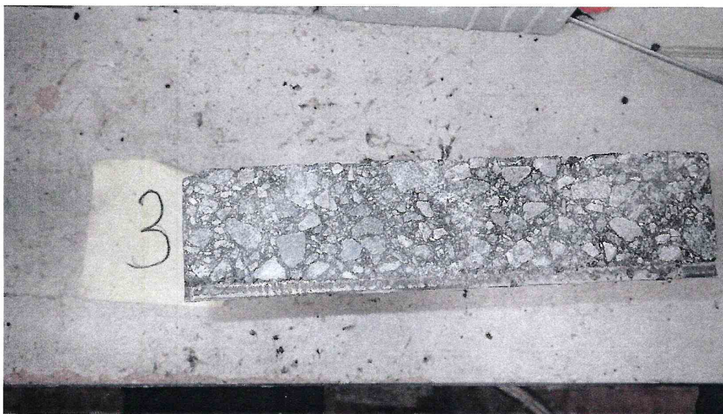
Рисунок 3 – Образец 16/7 МДС № 3, испытанный по ГОСТ Р 59180-2021. Определение прочности сцепления при сдвиге при температуре -40\text{ }^{\circ}\text{C}
