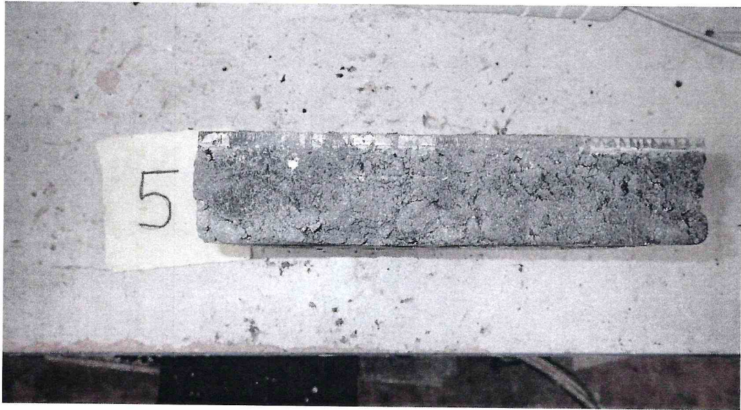
Рисунок 5 – Образец 16/7 МДС № 5, испытанный по ГОСТ Р 59180-2021. Определение прочности сцепления при сдвиге при температуре -40\text{ }^{\circ}\text{C}
