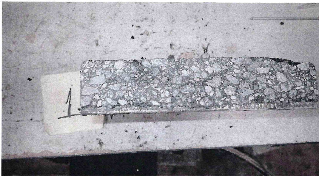
Рисунок 1 – Образец 16/7 МДС № 1, испытанный по ГОСТ Р 59180-2021. Определение прочности сцепления при сдвиге при температуре -40 °С
