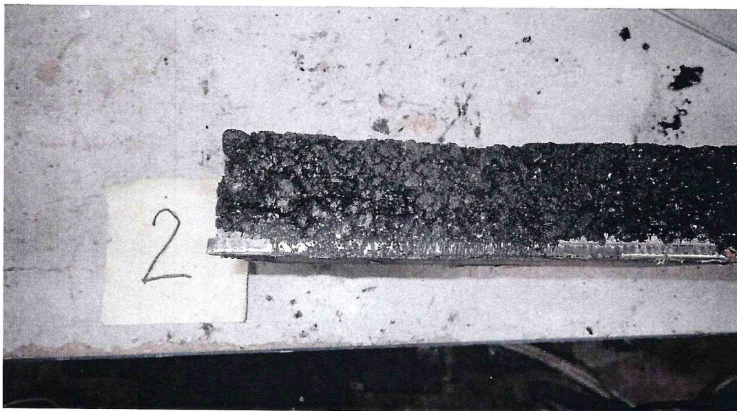
Рисунок 2 – Образец 16/8 МДС № 2, испытанный по ГОСТ Р 59180-2021. Определение прочности сцепления при сдвиге при температуре 50 °С
