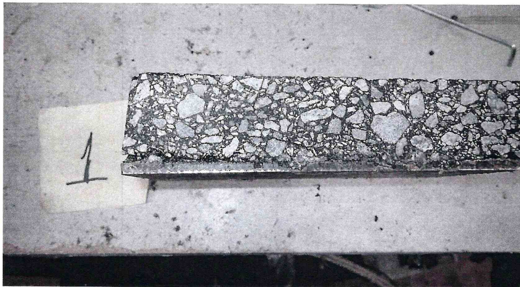
Рисунок 1 – Образец 16/8 МДС № 1, испытанный по ГОСТ Р 59180-2021. Определение прочности сцепления при сдвиге при температуре 50 °С
