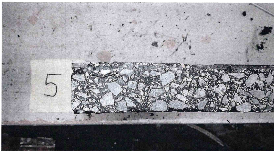
Рисунок 5 – Образец 16/8 МДС № 5, испытанный по ГОСТ Р 59180-2021. Определение прочности сцепления при сдвиге при температуре 50 °С
