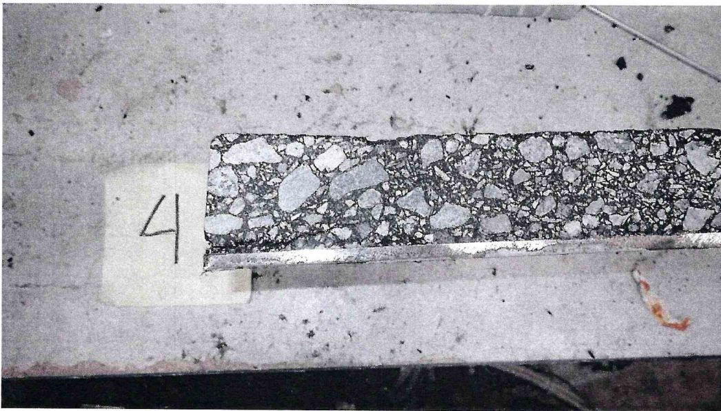
Рисунок 4 – Образец 16/8 МДС № 4, испытанный по ГОСТ Р 59180-2021. Определение прочности сцепления при сдвиге при температуре 50 °С
