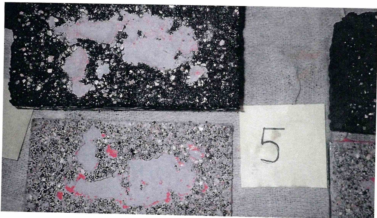
Рисунок 5 – Образец 210/5 МДС № 5, испытанный по ГОСТ Р 59180-2021. Определение прочности сцепления при сдвиге, при температуре -40\text{ }^{\circ}\text{C}
