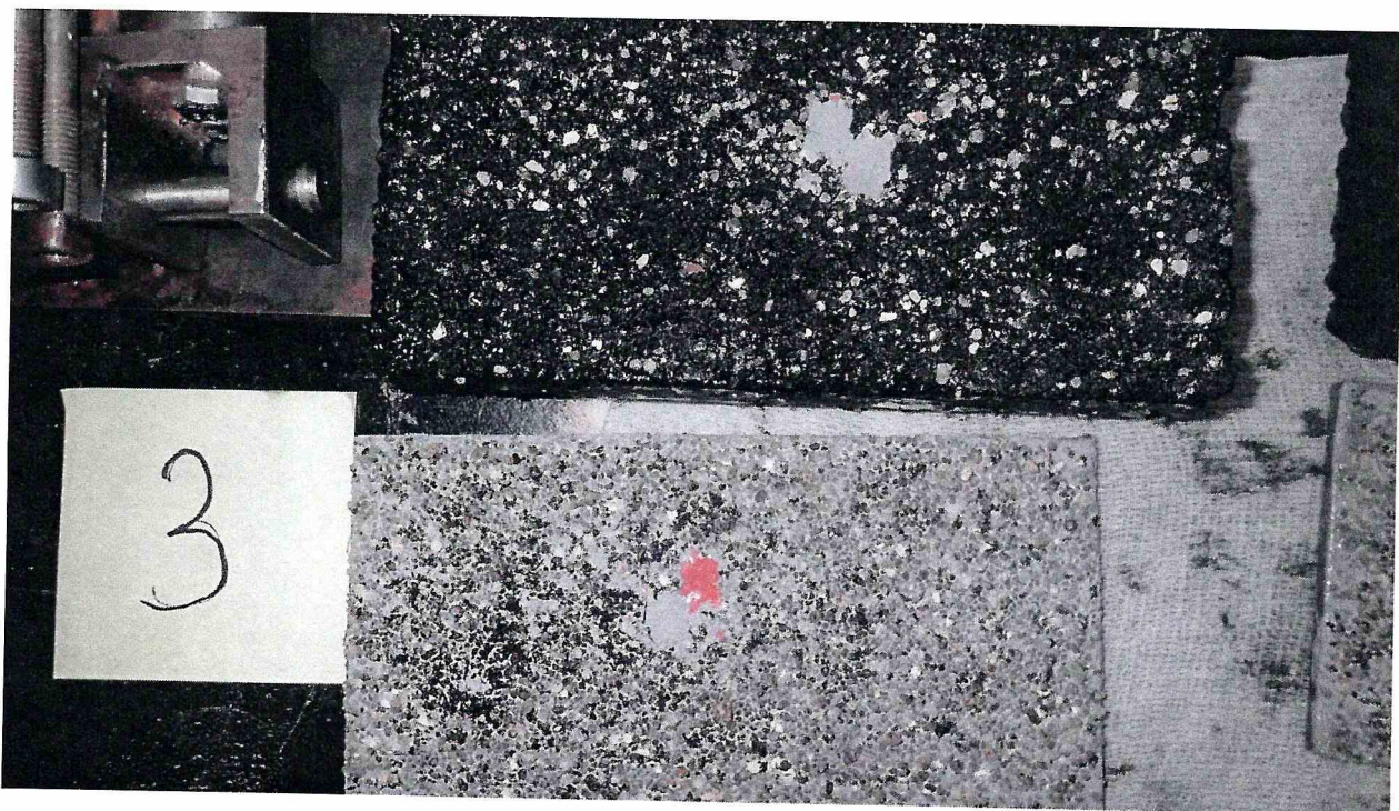
Рисунок 3 – Образец 210/5 МДС № 3, испытанный по ГОСТ Р 59180-2021. Определение прочности сцепления при сдвиге, при температуре -40\text{ }^{\circ}\text{C}
