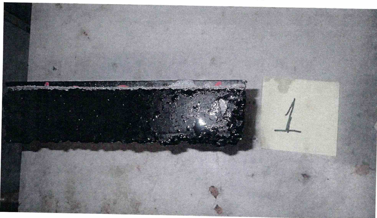
Рисунок 1 – Образец 210/5 МДС № 1, испытанный по ГОСТ Р 59180-2021. Определение прочности сцепления при сдвиге, при температуре -40 °С
